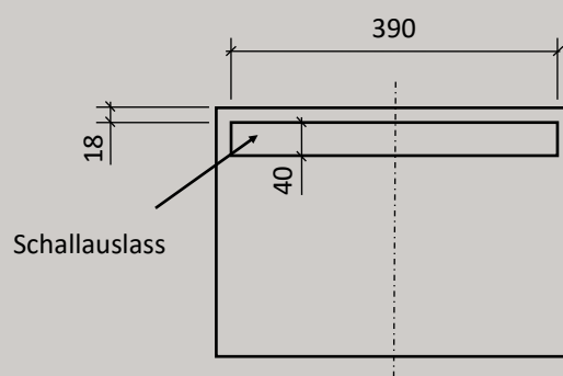
Untersicht
